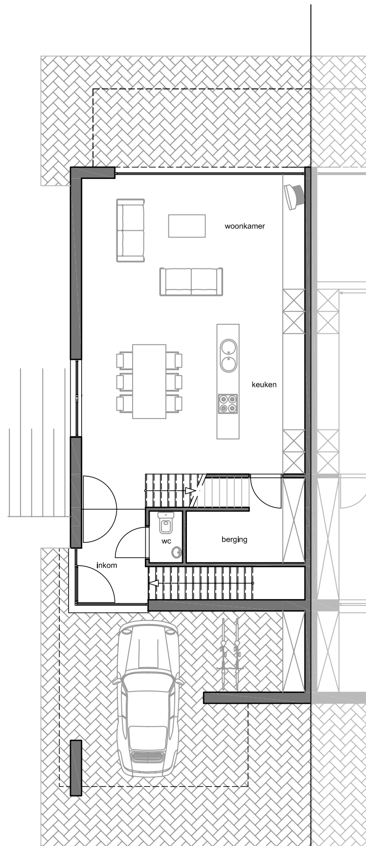
Blok B, woning 1: Plan gelijkvloers
