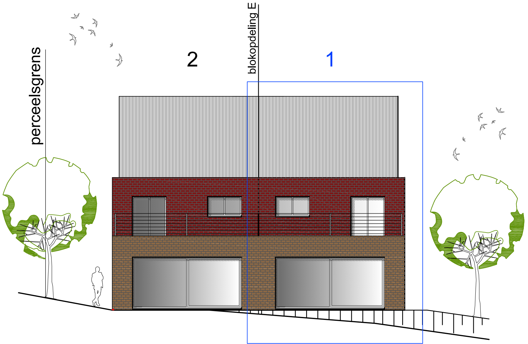
Blok E, woning 1 : Achtergevel
