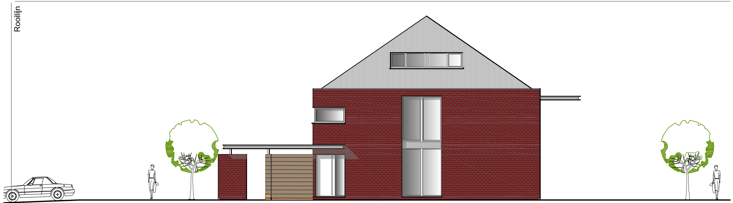
Blok D, woning 2 : Zijgevel rechts
