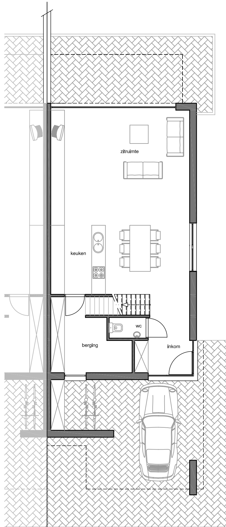
Blok D, woning 2: Plan gelijkvloers
