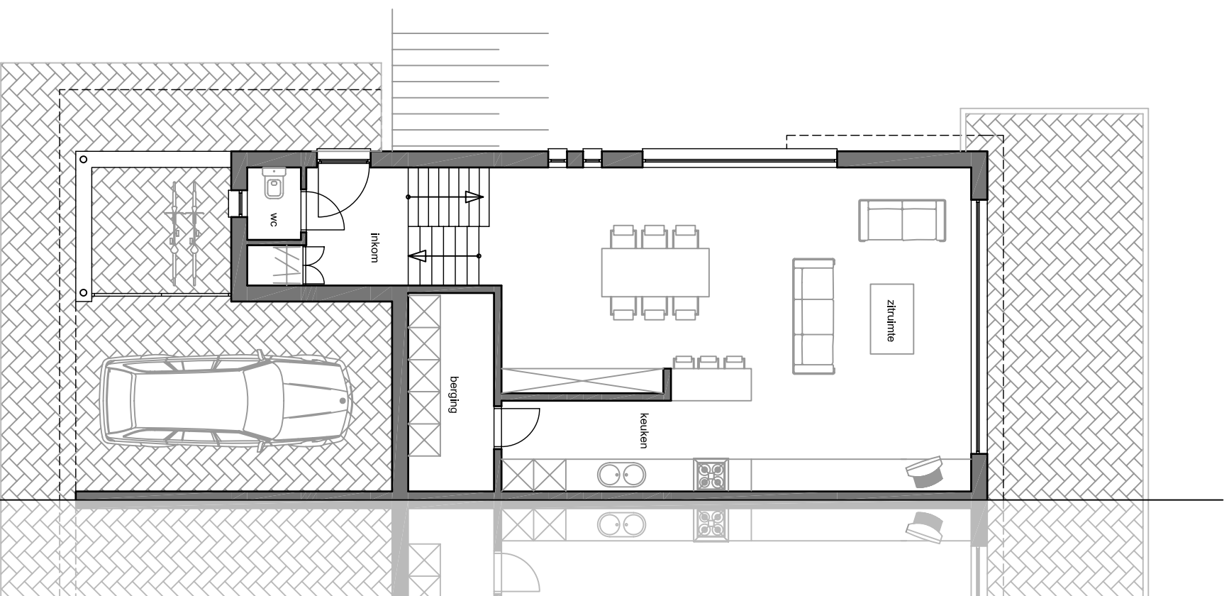
Blok C, woning 1: Plan gelijkvloers
