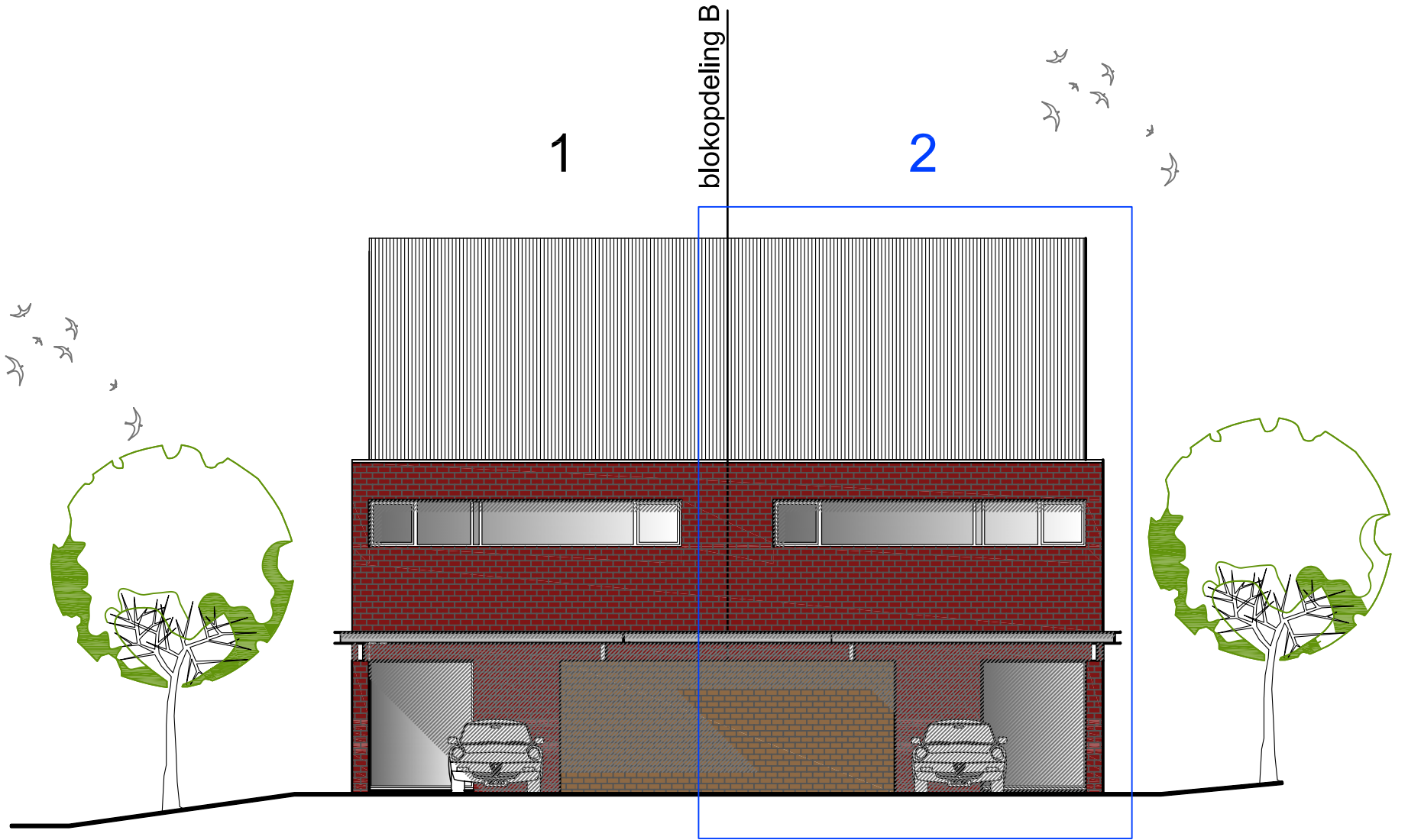
Blok B, woning 2 : Vorgevel
