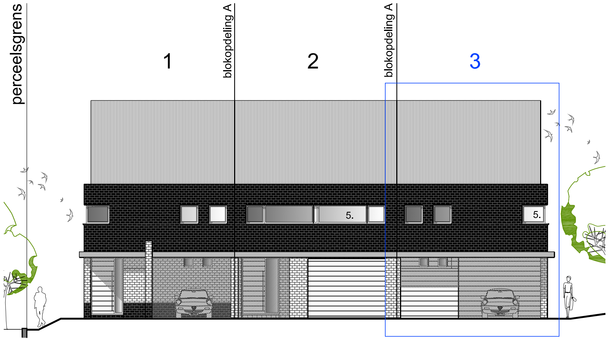
Blok A, woning 3 : Voorgevel
