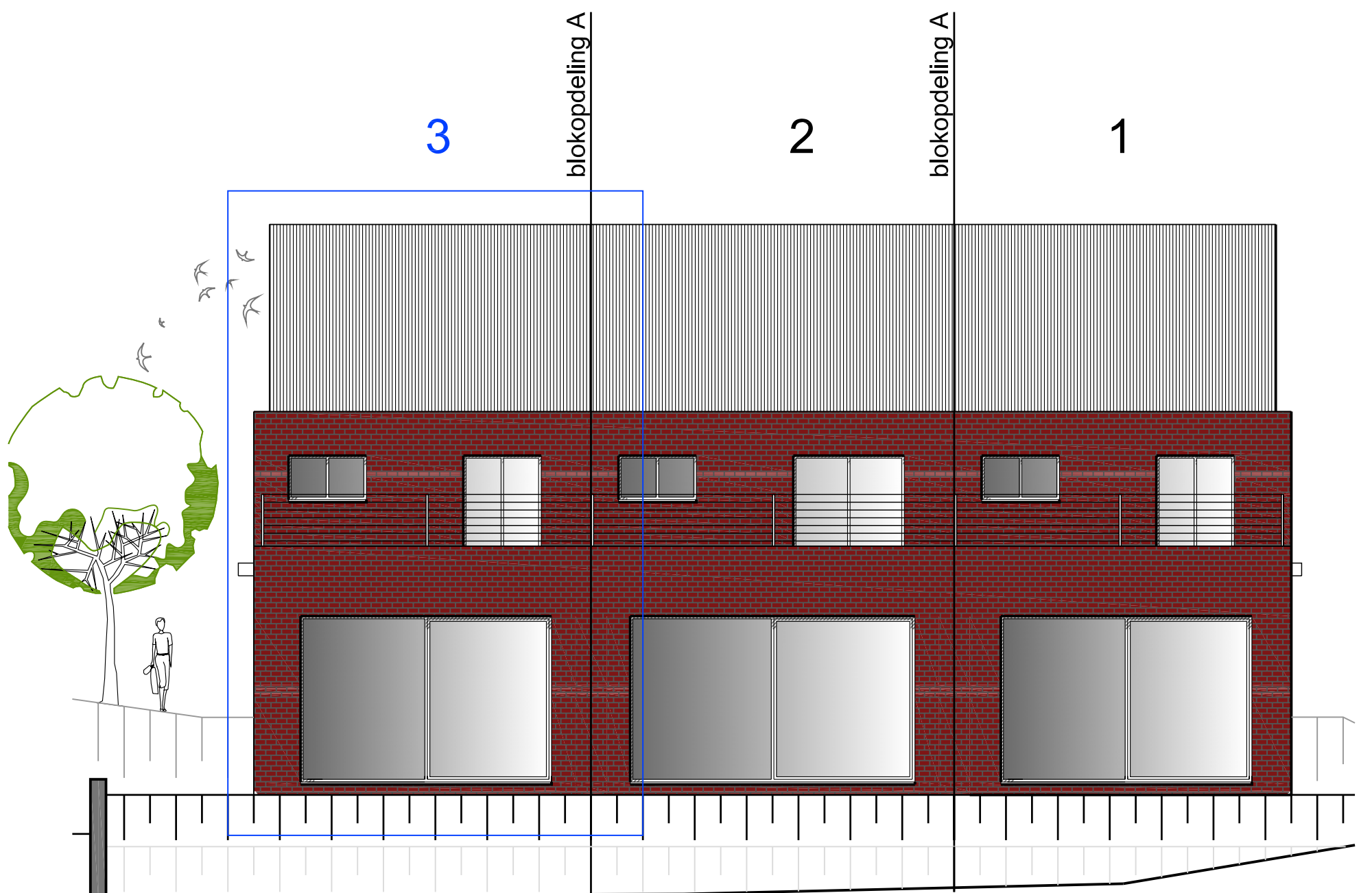
Blok A, woning 3 : Achtergevel
