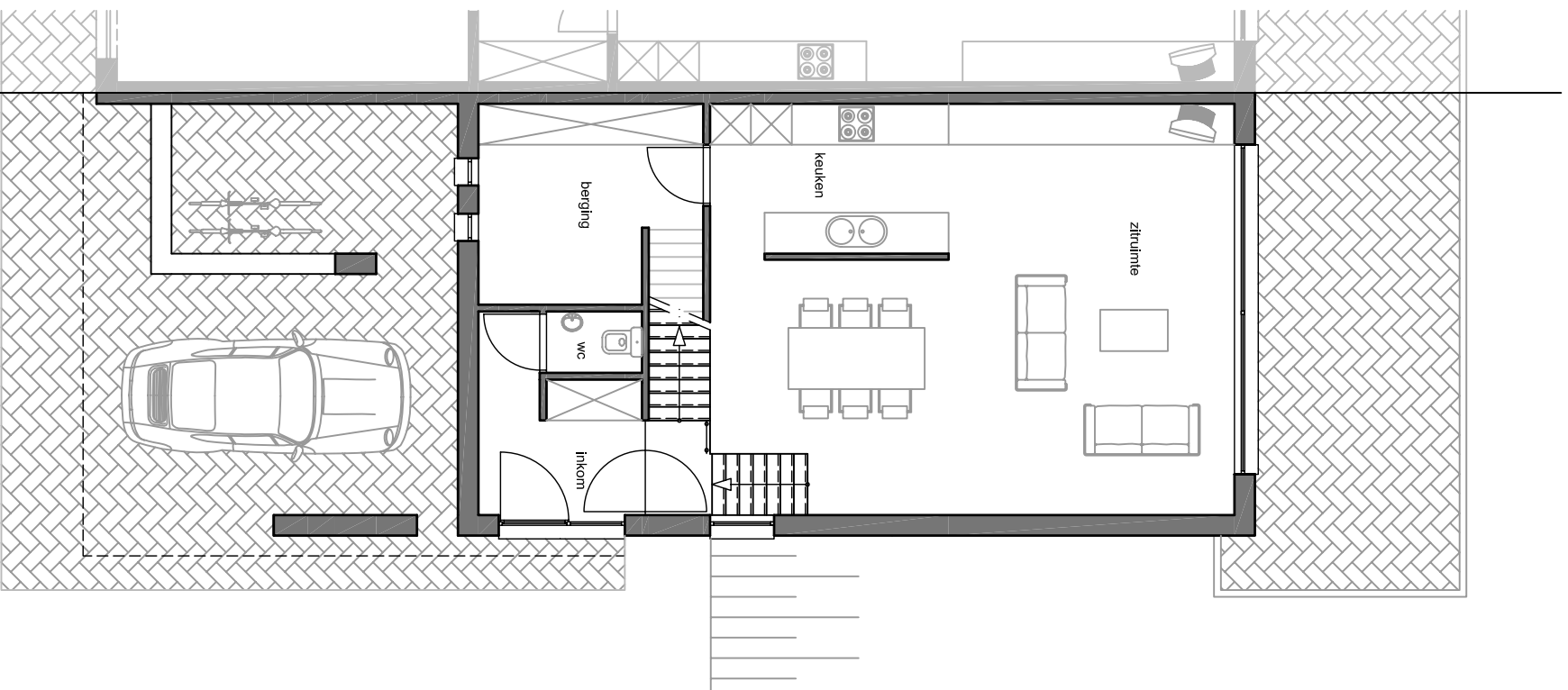
Blok A, woning 3: Plan gelijkvloers
