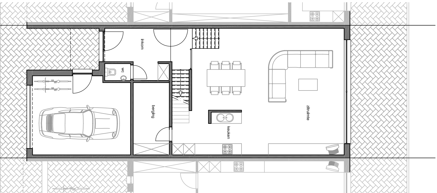
Blok A, woning 2: Plan gelijkvloers
