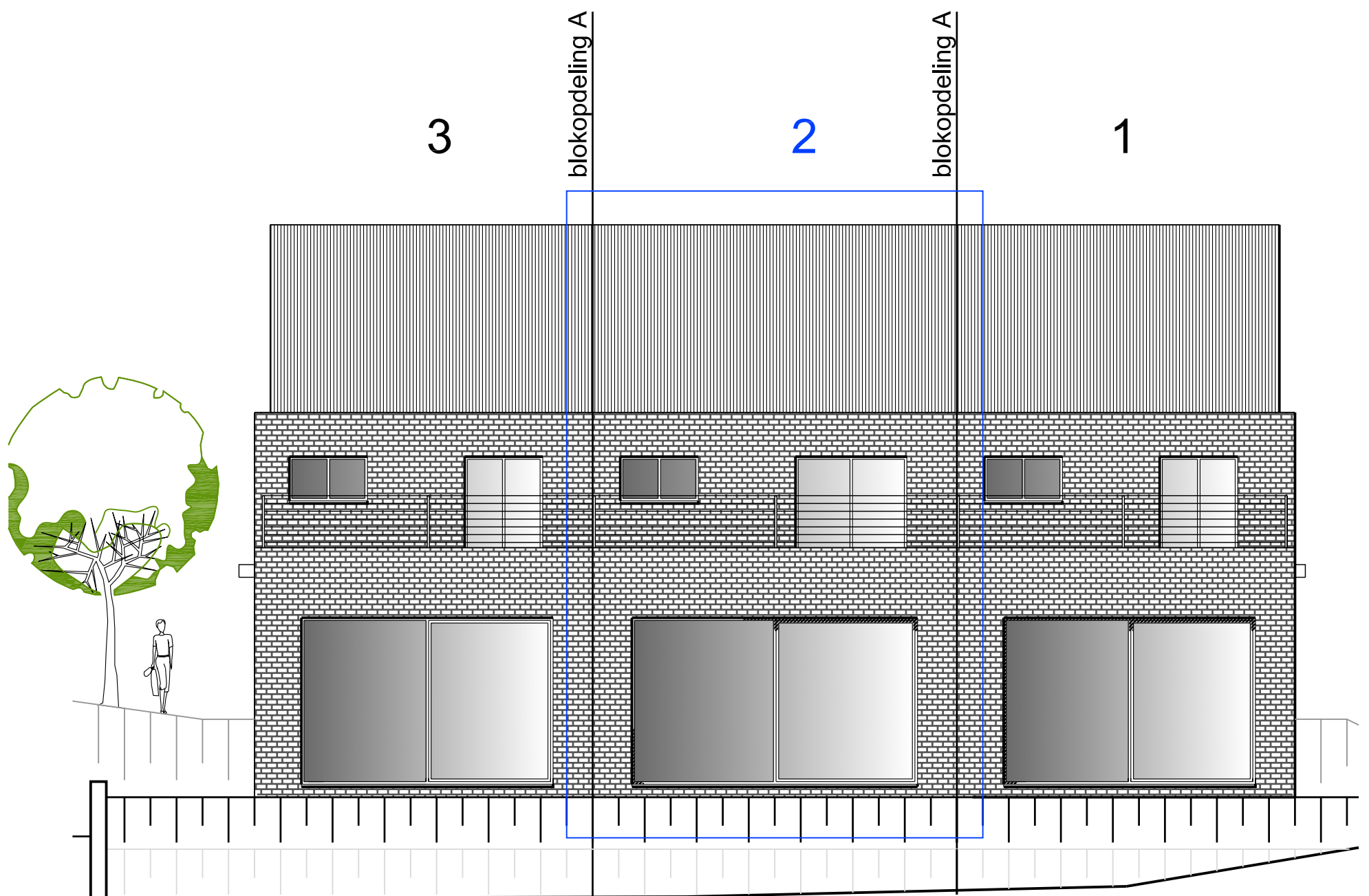
Blok A, woning 2 : Achtergevel
